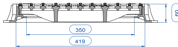
SEZIONE B-B
