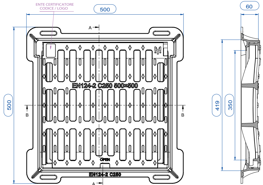
SEZIONE A-A
